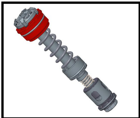
Bloc de compression
